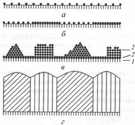
Рисунок 1.3 – Схема структурно-морфологічних перетворень за механізмом СК: a , b – структурні перетворення; c – утворення тривимірних острівців; d – полідоменна (полікристалічна) плівка. 1 – підкладка; 2' – двовимірне
