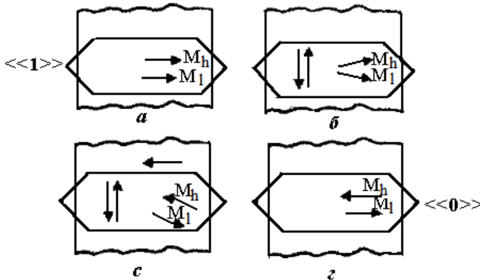
Рисунок 4.6 – Орієнтація векторів намагніченості \mathbf{M}_h і \mathbf{M}_l при поздовжньому розташуванні ВЛН: a , з – стани зберігання інформації; б , в – стани зчитування
