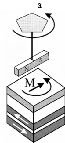
Рисунок 5.8 – Чутливі елементи ГМО - датчиків на основі багат шарової (а) та спін-вентильної (в) пліткових структур для детектування положення і повороту об'єкта. Залежність величини ГМО від товщини немагнітного прошарку Cu (б) та робоча характеристика датчика повороту (г)
