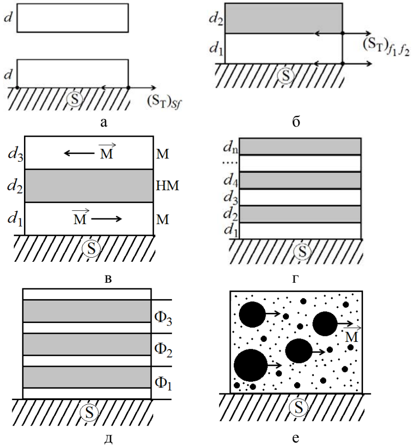
Рисунок 1.4 – Типи плівкових наноструктур: одношарова плівка у вільному стані або на підкладці (а); двошарова система (б); тришарова система (в); багатошарова
