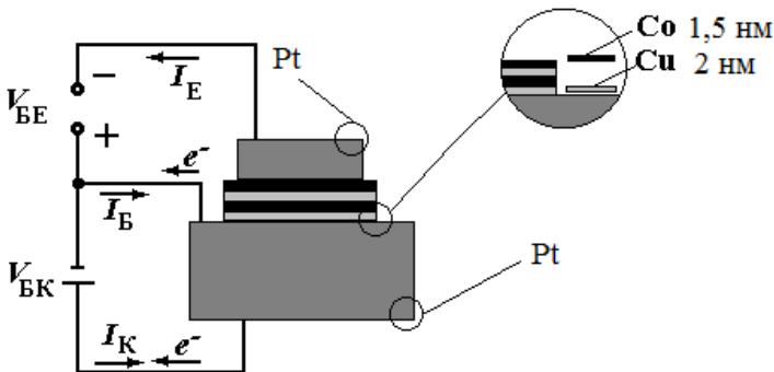
Рис. 5.5. Структура СВ-транзистора на гарячих електронах: V_{BE} – напруга база-емітер; V_{BK} – колекторно-
