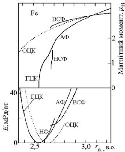
Рисунок 2.2 – Залежність магнітного моменту і загальної магнітної енергії взаємодії для ГЦК-Fe (суцільна лінія) і ОЦК-Fe (пунктирна лінія) від міжатомної відстані: НМ – немагнітна фаза; АФ – антиферромагнетик; НСФ – низько-спіновий феромагнетик; ВСФ – високоспіновий феромагнетик. Рд – одиниця вимірювання енергії резерфорд
