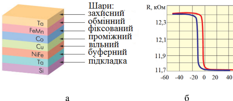
Рисунок 3.4 – Приклад структури спін-вентилля (а) та його робочої характеристики (б)
