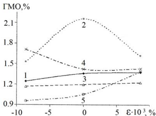
Рисунок 5.12 – Залежність величини ГМО від поздовжньої деформації для псевдоспін-вентилів \text{Cr}(5\text{нм})/\text{Au}(2,5\text{нм})/\text{Co}(5\text{нм})/\text{Au}(d\text{нм})/\text{Co}(2\text{нм}) для різних товщин плівки Au, нм: 1 – 2,2; 2 – 2,4; 3 – 2,9; 4 – 3,3 та 5 – 4,0
