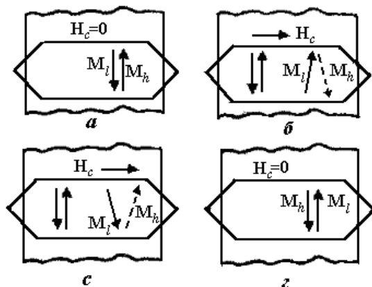
Рисунок 4.7 – Орієнтація векторів намагніченості \mathbf{M}_h і \mathbf{M}_l при поперечному розташуванні ВЛН: a , г – стани зберігання інформації; б , в – стани зчитування
