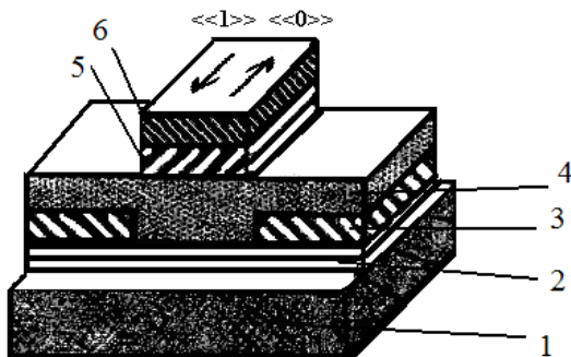
Рисунок 4.8 – Структура комірки СВЗЕ зі статичним зчитуванням, з розділеними областями зберігання і
