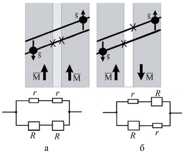
Рисунок 3.3 – Механізм виникнення ГМО на межі поділу шарів ФМ/ІМ і ІМ/ФМ та відповідні еквівалентні схеми провідності по низькоомному ( r + r ) та високоомному ( R + R ) спінових каналах: феромагнітна (а) та антиферомагнітна (б) орієнтації магнітних моментів
