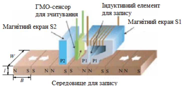
Рисунок 5 – ГМО-головка жорсткого диска (із праці Чапперта та ін. [18])
