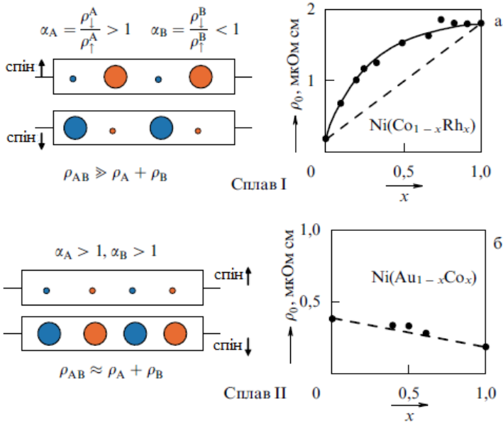
Рисунок 2 – Експерименти, що проведені на трикомпонентних сплавах із використанням аналогічного з ГМО принципу [4]: а - схематичне зображення спін-
