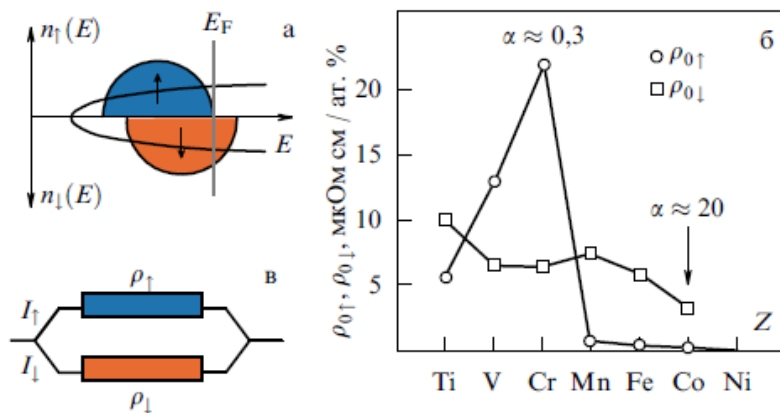
Рисунок 1 – Основи спітроніки: а - схематичне зображення зонної структури ферромагнітного металу, що відображає розщеплення енергетичних зон з урахуванням орієнтації спінів; б - опори спінових каналів провідності (в
