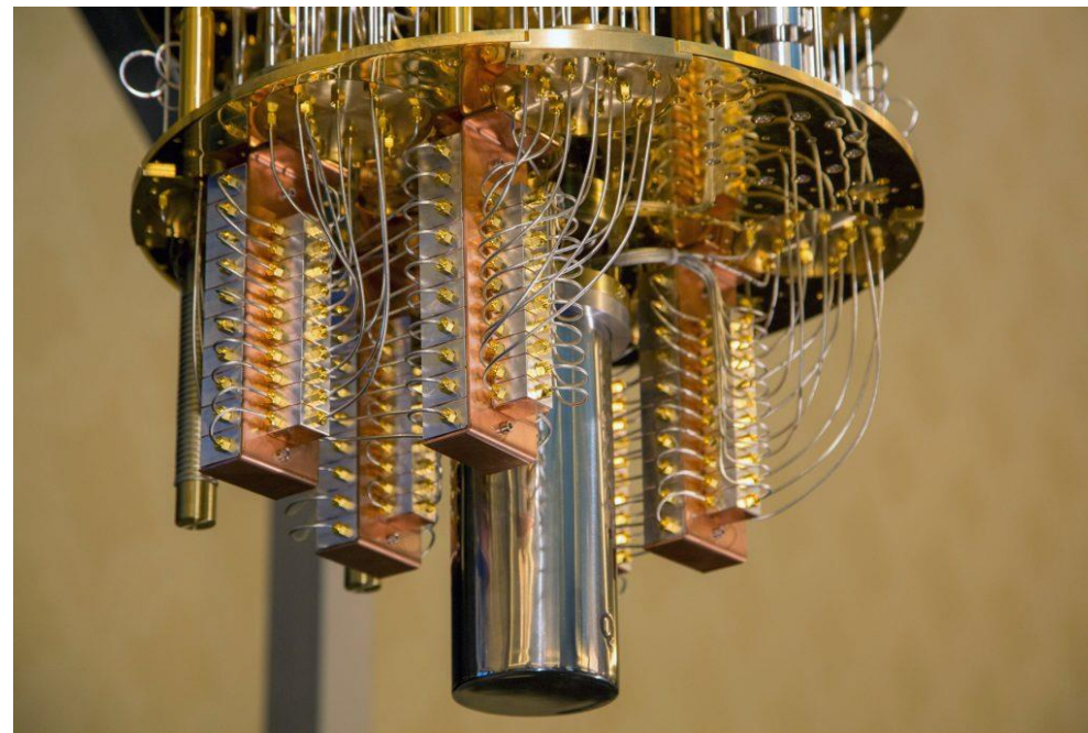
50-ти кубітний процесор Intel
