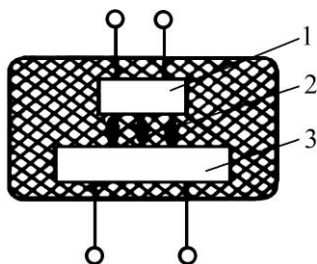
Рисунок 8.1 - Принцип будови оптопари: 1 - випромінювач, 2 - оптичний прозорий клей, 3 - фотоприймач
