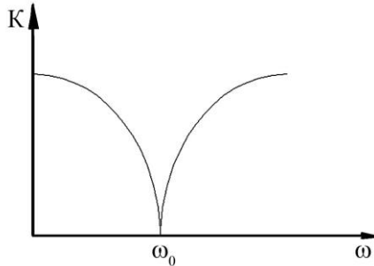
Рисунок 4.6 – Характеристика RC-нульового фільтра ІМС
