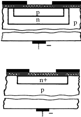
Рисунок 3.13 - Дифузійні резистори НІМС: р-типу (а), n-типу (б)
