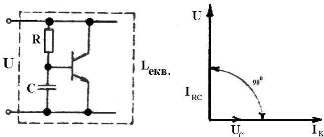
Рисунок 3.15 - Еквівалент індуктивності
