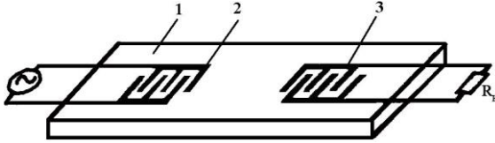
Рисунок 6.13 - Принцип будови акустoeлектронного приладу на поверхневих акустичних хвилях
