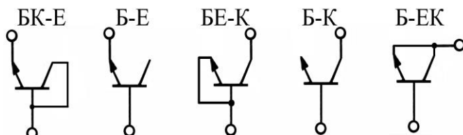
Рисунок 3.12 - Варіанти використання транзисторів у діодному ввімкненні
