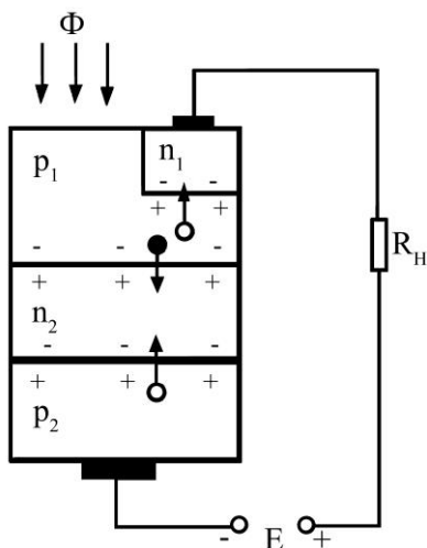
Рисунок 6.19 - Структура фототиристора
