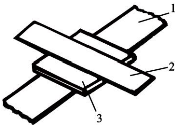
Рисунок 6.22 - Плівковий кріотрон
