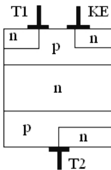
Рисунок 7.8 – Структура симістора
