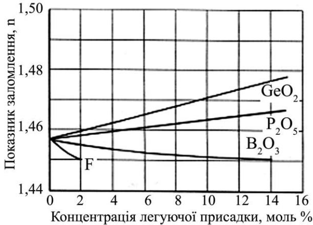
Рисунок 9.1 - Показники заломлення кварцового скла з різними легуючими присадками
