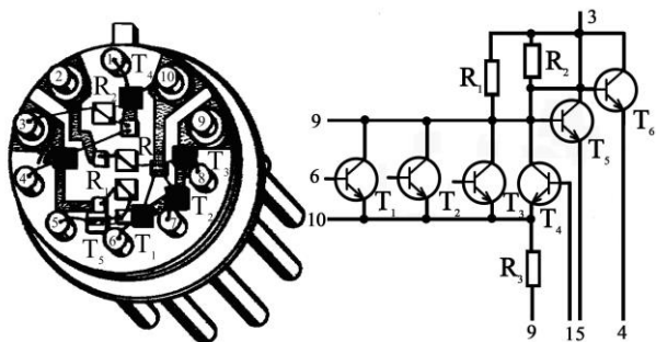
Рисунок 3.3 - Структура та електрична схема багатокристалльної НІМС
