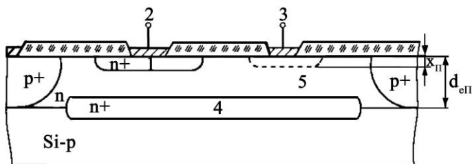
Рисунок 2.4 - Структура діода Шотткі
