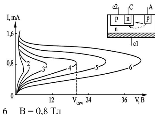
Рисунок 6.12 – ВАХ Si- магніотиристиора, відстань між p-областями 100 мкм: 1 – B = -1 \text{ Тл} ; 2 – B = -0,8 \text{ Тл} ; 3 – B = -0,4 \text{ Тл} ; 4 – B = 0 ; 5 – B = 0,4 \text{ Тл} ;
