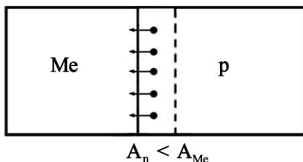
Рисунок 2.3 - Контакт металу з напівпровідником p-типу
