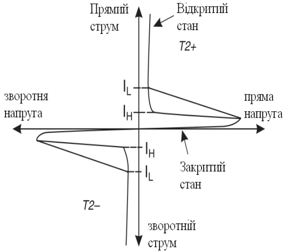
Рисунок 7.9 – Вольт-амперна характеристика симістора
