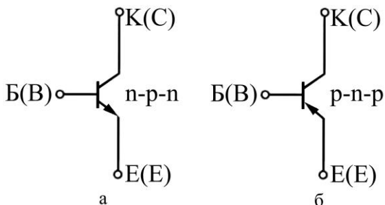
Рисунок 3.8 – Графічне позначення БТ
