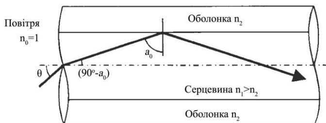
Рисунок 9.2 – Хід променів в оптоволокну. \alpha_0 - кут повного відзеркалення
