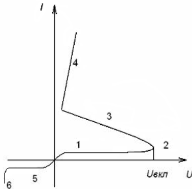
Рисунок 7.5 – Вольт-амперна характеристика діністора:
