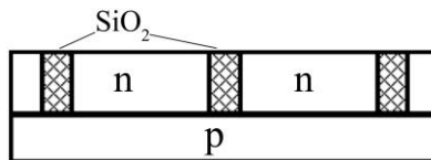
Рисунок 3.6 - Комбінована ізоляції
