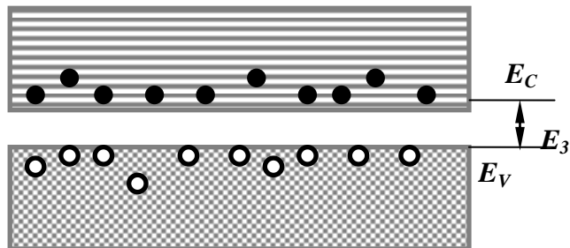
Рисунок 2.1 - Валентна зона (білі кружечки - дірки) та зона провідності (чорні кружечки-електрони провідності): E_g -ширина забороненої зони; E_C -дно зони провідності; E_V - потолок валентної зони
